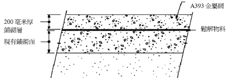
詳圖 1:20 B
