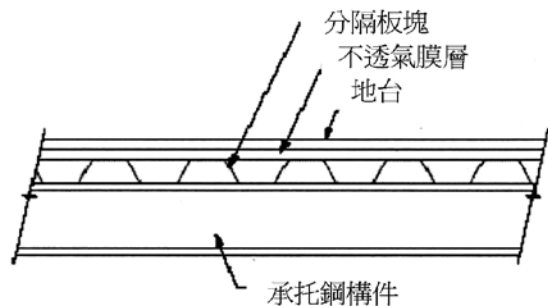
詳圖 1:20 A
